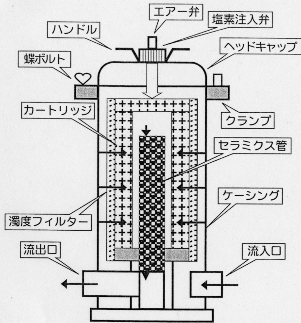
Well-Q21-400W浄水器の仕様
